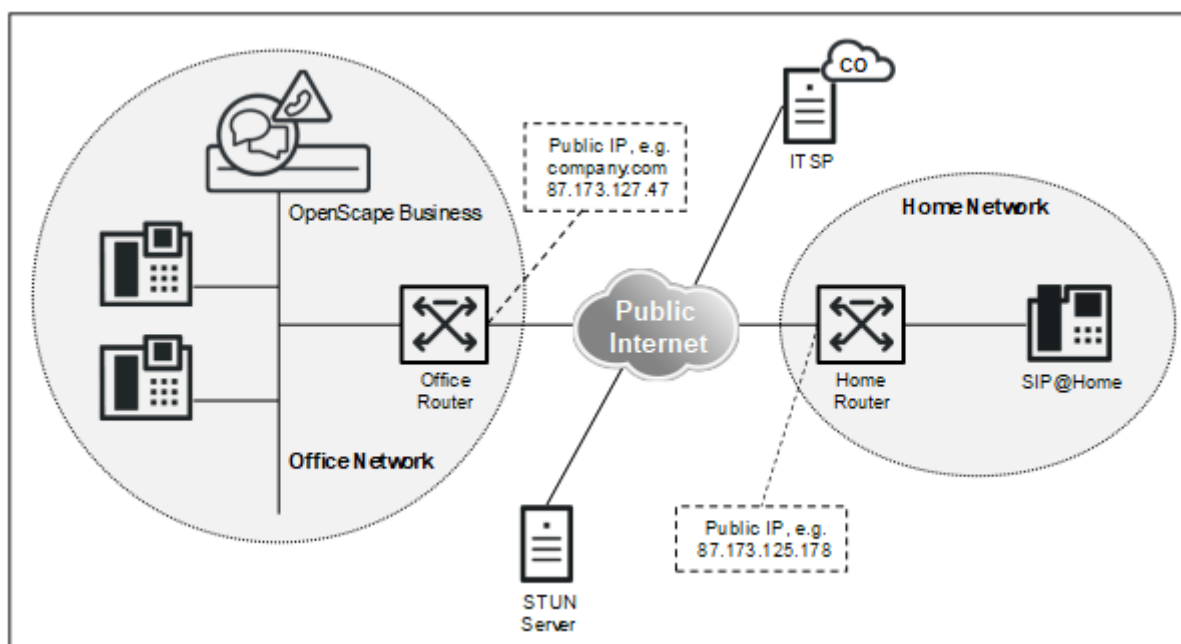
Illustration 7 : Composantes d'Equipement@Home (Equipement SIP@Home ou Equipement Système@Home)
